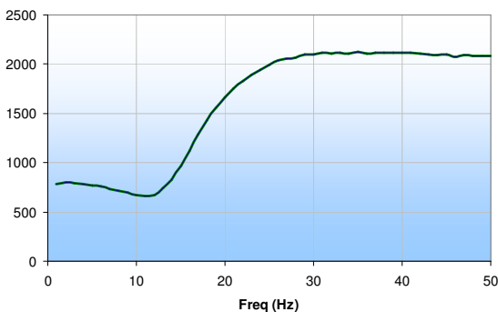
Dynamic stiffness Y 0.1mm
