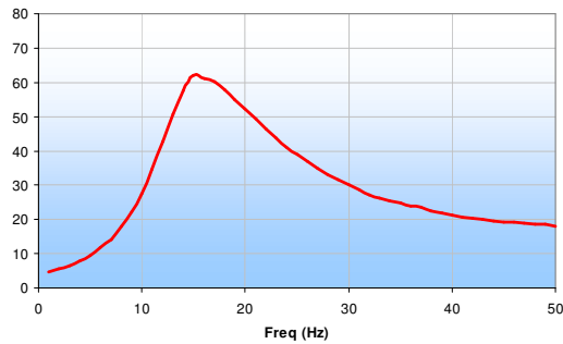
Dynamic stiffness Y 0.1mm
